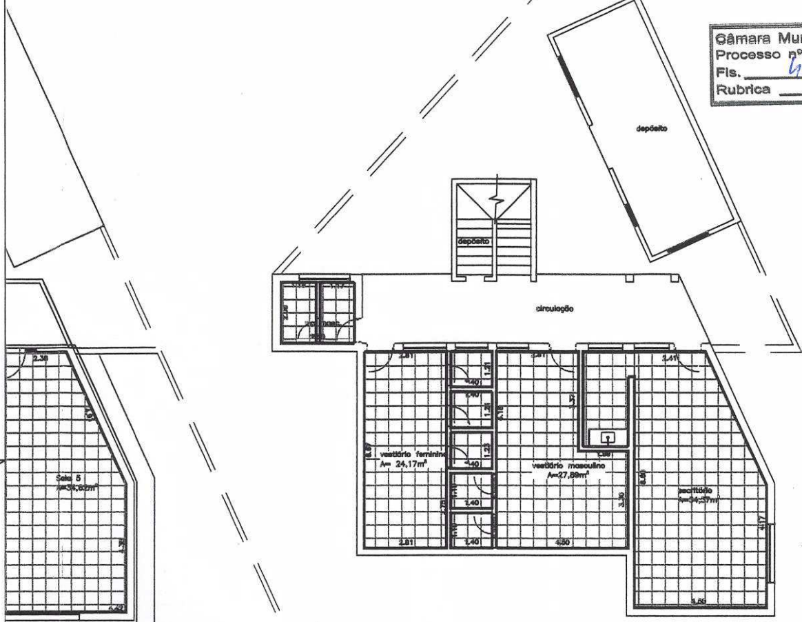
Planta baixa pav. inferior escala 1:100
