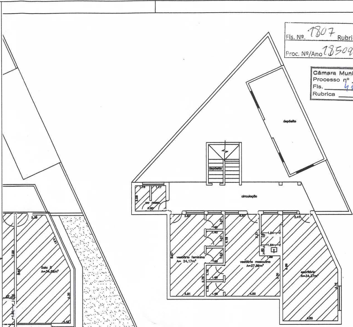
Planta baixa pav. inferior escala 1:100
